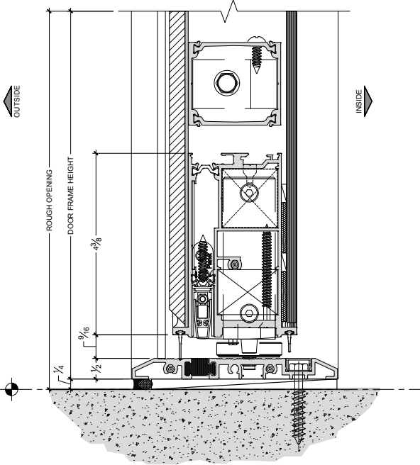
1 SECTION DETAIL - ES-PSD5030T - SILL OPTION 1 SCALE: 6" - 0" = 1' - 0"
