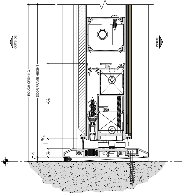
2 SECTION DETAIL - ES-PSD5030T - SILL OPTION 2 SCALE: 6" - 0" = 1' - 0"
